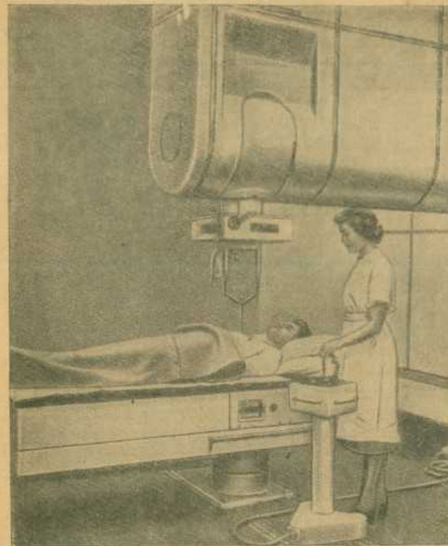
Рис. 43. Английский линейный электронный ускоритель на энергию 8 Мэв для рентгенотерапии.
