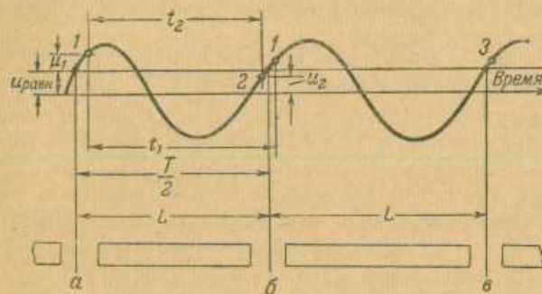
Рис. 12. Автофазировка в линейном ускорителе с пролетными трубками.
