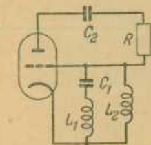
Рис. 25. Схема автогенератора 6-метрового фазотрона.
