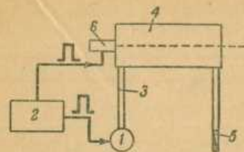
Рис. 17. Блок-схема высокочастотного устройства линейного ускорителя с бегущей волной.
