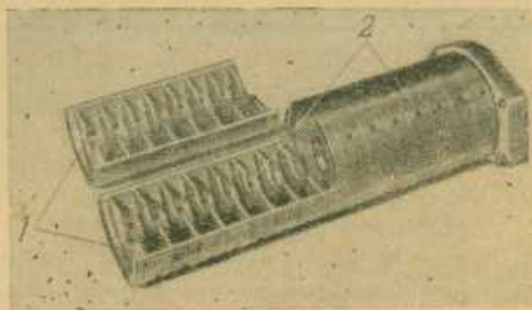
Рис. 16. Основной узел линейного ускорителя с бегущей волной — диафрагмированный волновод. 1 — диафрагмы; 2 — отверстия для откачки волновода.
