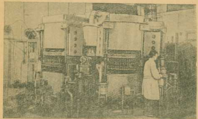
Рис. 31. Синхротрон на 265 Мэв Физического института имени Лебедева Академии наук СССР.
