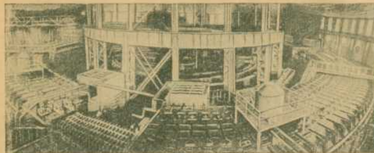
Рис. 33. Общий вид синхрофазотрона на 10 млрд. эв Объединенного Г института ядерных исследований (СССР).
