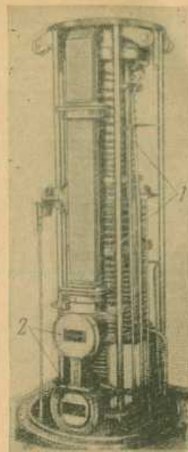
Рис. 18. Устройство английского линейного ускорителя с бегущей волной.
