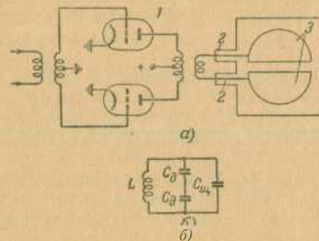
Рис. 22. Упрощенная схема оконечного каскада высокочастотного усилителя циклотрона. 1 — оконечный каскад генератора высокой частоты; 2 — линии; 3 — дуанты.
