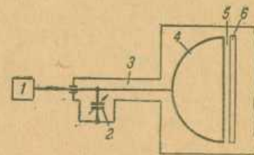
Рис. 24. Блок-схема высокочастотного устройства 6-метрового фазотрона.
