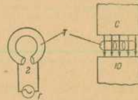
Рис. 10. Принципиальная схема ускорения частиц малым переменным напряжением в присутствии магнитного поля (циклическое ускорение). T — трубка; G — генератор.
