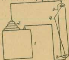
Рис. 4. Схема ускорителя с постоянным напряжением (масштабы на рисунке не соблюдены).
