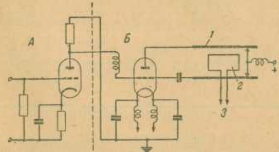
Рис. 30. Схема автогенератора для синхротрона на 35 Мэв.
