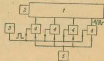
Рис. 13. Блок-схема высокочастотного устройства линейного ускорителя с протонными трубками.
