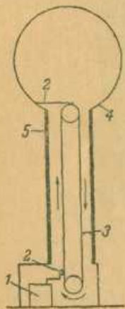
Рис. 7. Схема электростатического генератора Ван де Граафа.
