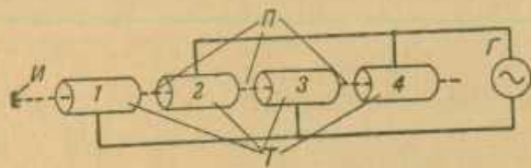
Рис. 9. Принципиальная схема ускорения частиц малым переменным напряжением (линейное ускорение).
